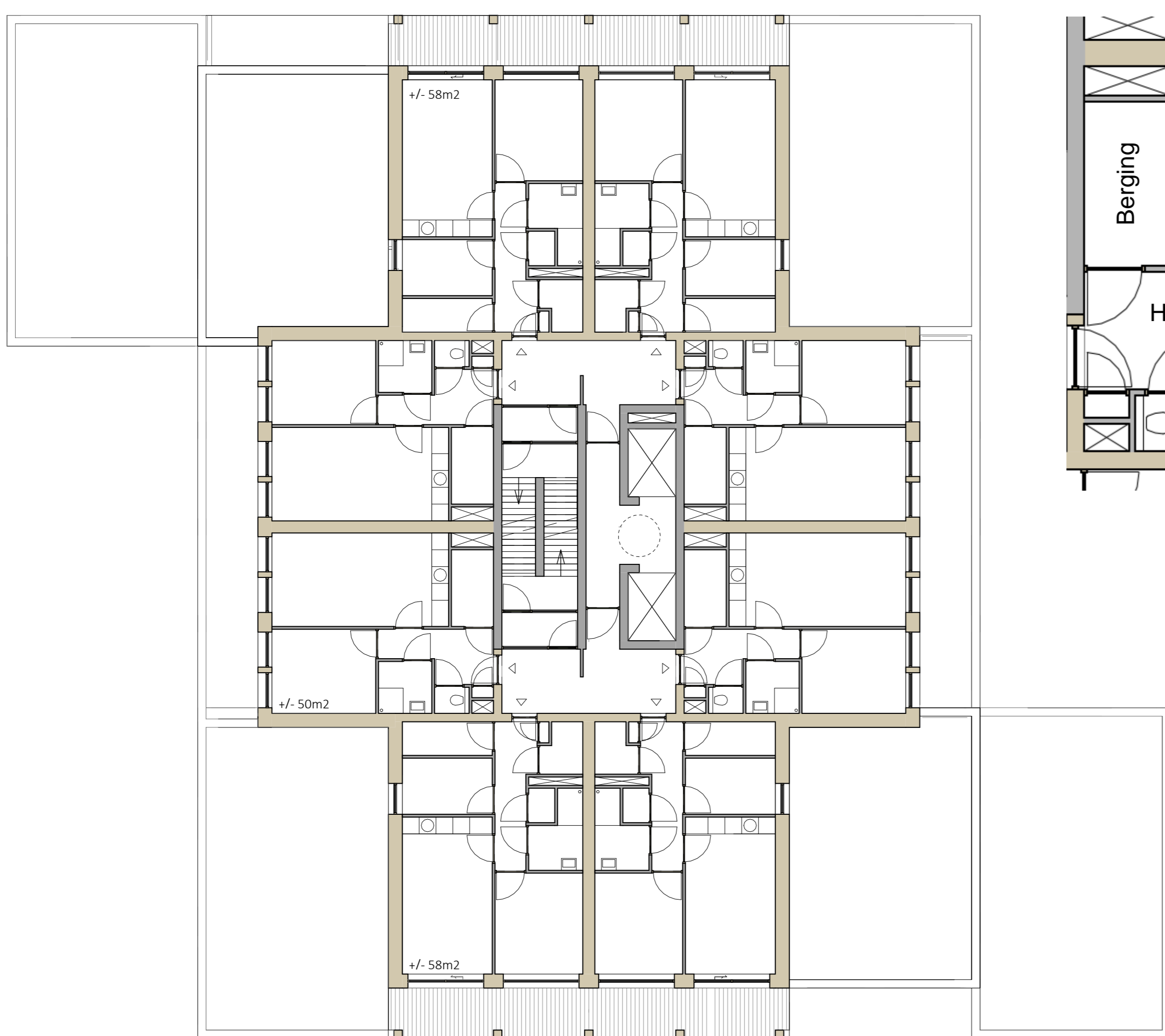
Concept gebouwstructuur & plattegronden
